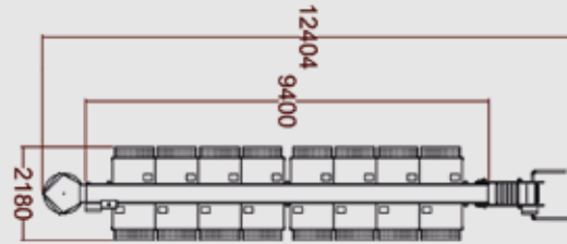
Üst Görünüm / Top View
