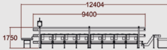
Yan Görünüm / Side View
